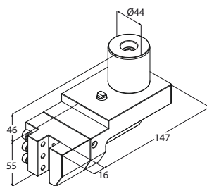
Portautensile
