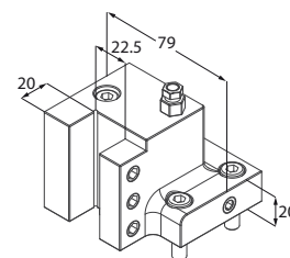
Portautensile
