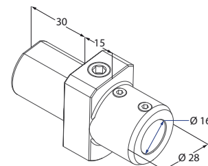
Portabareno
