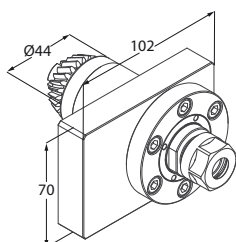
Motorizzato assiale
