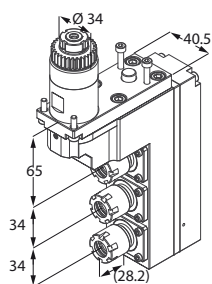
Motorizzato triplo
