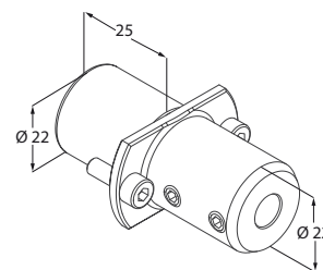
Portabareno
