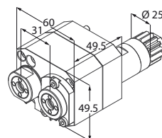
Motorizzato radiale moltiplicatore di giri
