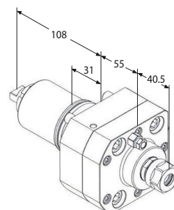
Motorizzato assiale
