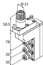
Motorizzato triplo fronte/retro
