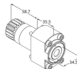
Motorizzato porta fresa
