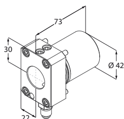
Portabareno
