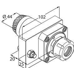
Motorizzato radiale
