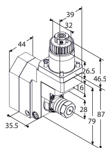
Motorizzato porta fresa a disco
