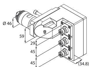
Motorizzato assiale triplo
