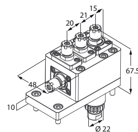
Motorizzato triplo
