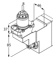
Motorizzato trasversale
