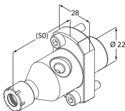
Porta punta
