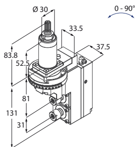
Motorizzato assiale doppio
