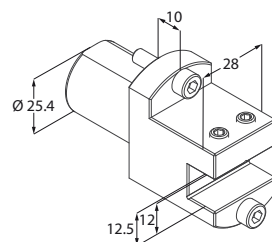
Portautensile
