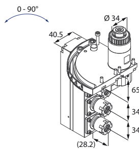
Motorizzato triplo
