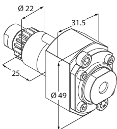
Portafresa
