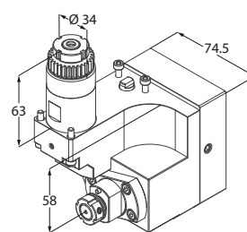
Motorizzato porta fresa
