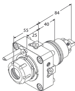
Motorizzato radiale
