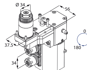
Motorizzato doppio
