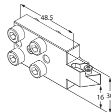
Portautensile a tornire
