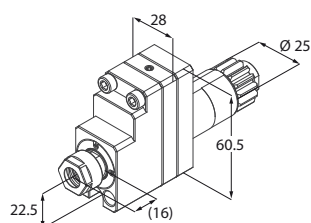
Motorizzato radiale
