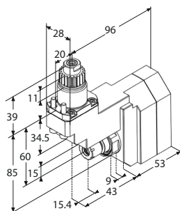
Motorizzato radiale
