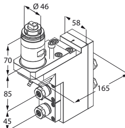
Motorizzato doppio
