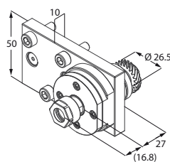
Motorizzato assiale
