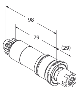
Motorizzato assiale
