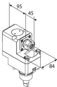
Motorizzato assiale
