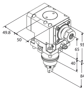
Motorizzato assiale
