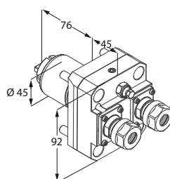
Motorizzato assiale doppio
