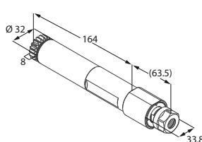
Motorizzato trasversale
