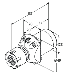
Portautensile fisso
