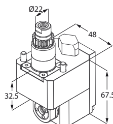
Motorizzato trasversale
