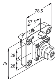
Motorizzato assiale
