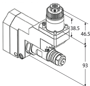
Motorizzato porta fresa a disco
