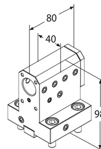
Portabareno
