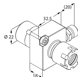
Portapunta con refrigerazione interna
