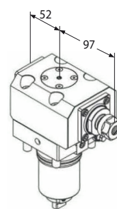
Motorizzato radiale
