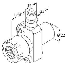
Portapunta con refrigerazione interna
