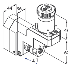
Motorizzato radiale e assiale
