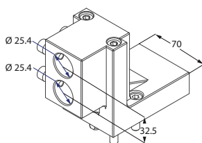
Portabareno doppio
