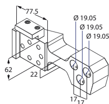
Portabareno triplo
