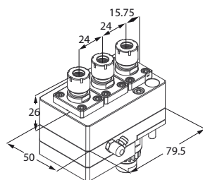
Motorizzato triplo
