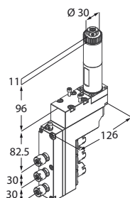
Motorizzato assiale triplo
