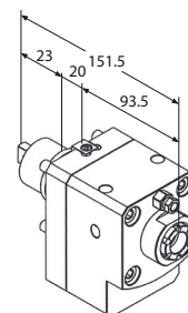
Motorizzato radiale
