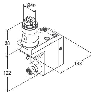
Motorizzato porta fresa a disco
