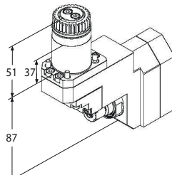
Motorizzato radiale
