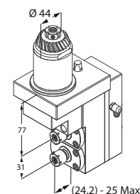
Motorizzato radiale
