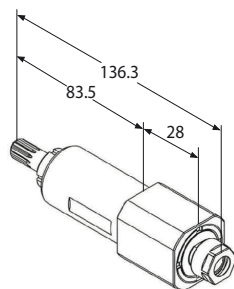
Motorizzato radiale e assiale
