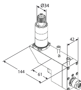
Motorizzato assiale
