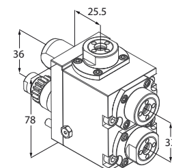
Motorizzato radiale e assiale
