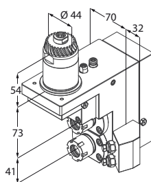
Motorizzato assiale doppio
