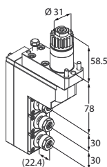
Motorizzato triplo
