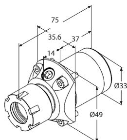
Portautensile fisso
