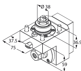
Motorizzato radiale
