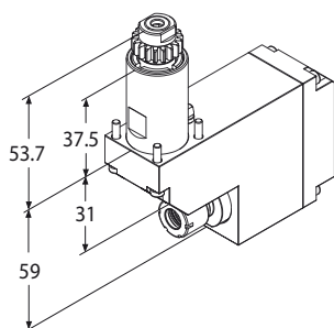
Motorizzato assiale
