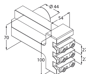
Portautensile triplo
