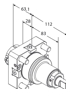
Motorizzato radiale
