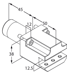
Portautensile
