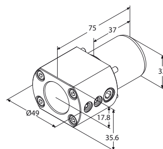
Portabareno
