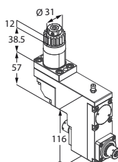
Motorizzato singolo
