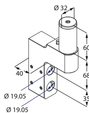
Portabareno
