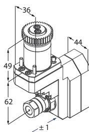
Motorizzato porta fresa a disco
