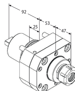
Motorizzato assiale
