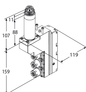
Motorizzato assiale triplo
