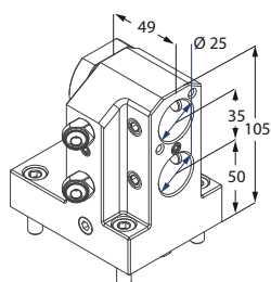
Portabareno doppio
