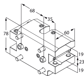
Portautensile doppio
