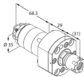
Motorizzato trasversale
