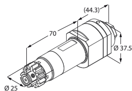
Motorizzato trasversale
