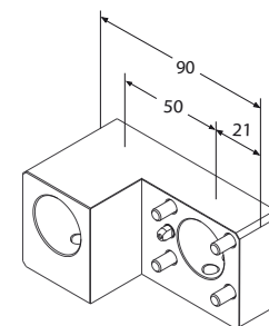
Portabareno doppio
