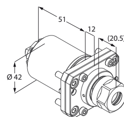
Motorizzato singolo
