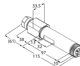
Motorizzato radiale
