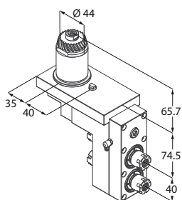
Motorizzato assiale doppio
