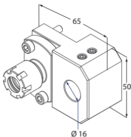
Estensione per portautensile
