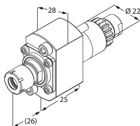
Motorizzato singolo
