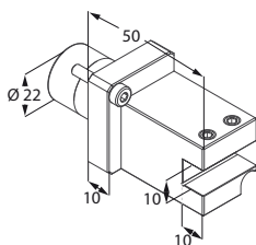
Portautensile
