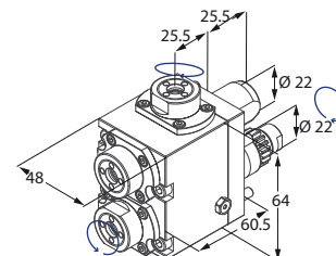
Motorizzato trasversale e frontale
