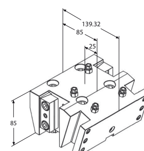
Portautensile fisso
