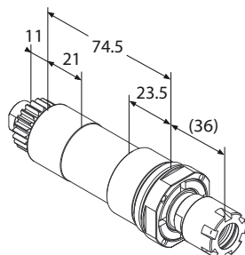
Motorizzato radiale
