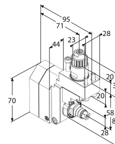
Motorizzato porta fresa a disco
