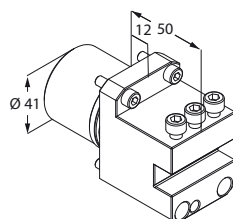
Portautensile
