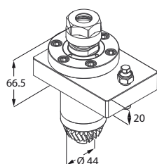
Motorizzato assiale
