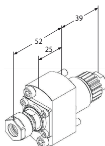
Motorizzato radiale e assiale
