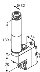
Motorizzato singolo
