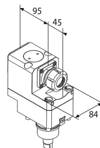
Motorizzato assiale
