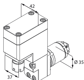
Motorizzato trasversale
