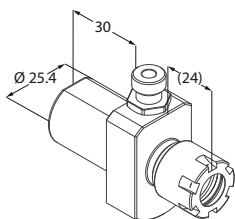
Porta pinza ER
