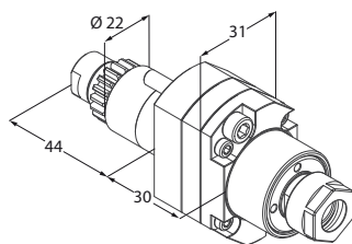
Moltiplicatore di giri
