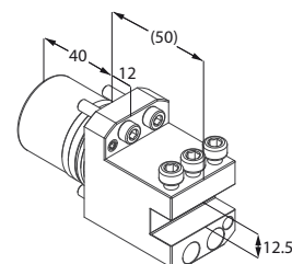
Portautensile
