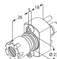
Porta punta (per foratura profonda)
