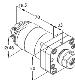
Motorizzato trasversale
