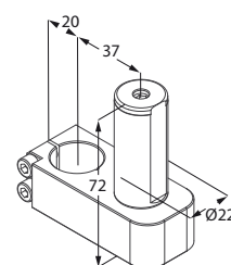
Portautensile ad aria
