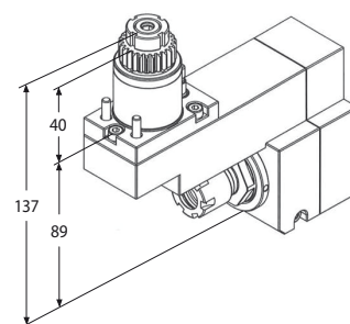
Motorizzato assiale
