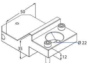
Portabareno
