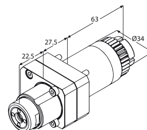
Motorizzato radiale
