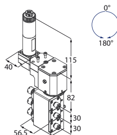
Motorizzato assiale triplo orientabile
