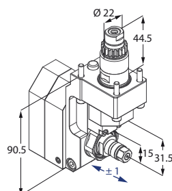
Motorizzato porta fresa
