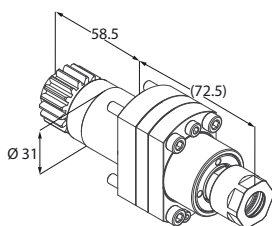
Motorizzato radiale moltiplicatore di giri
