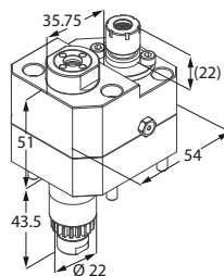
Motorizzato doppio
