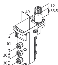
Motorizzato triplo
