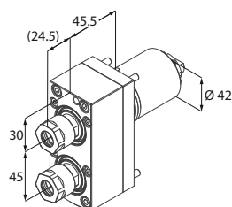
Motorizzato radiale doppio
