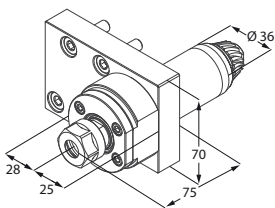
Motorizzato assiale
