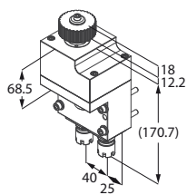
Motorizzato trasversale doppio
