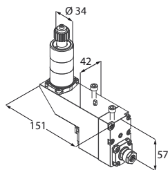
Motorizzato assiale
