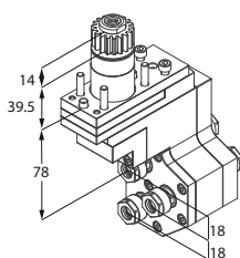
Motorizzato triplo
