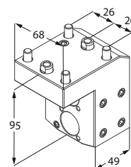
Portabareno
