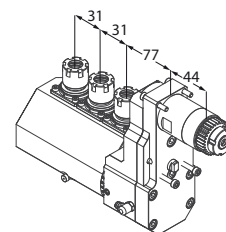
Motorizzato triplo
