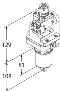
Motorizzato radiale
