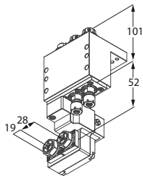
Motorizzato quadruplo
