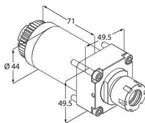
Motorizzato radiale
