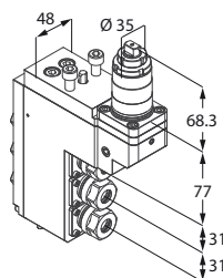
Motorizzato triplo
