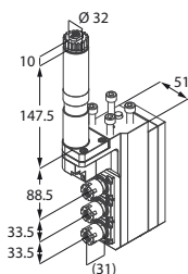
Motorizzato triplo
