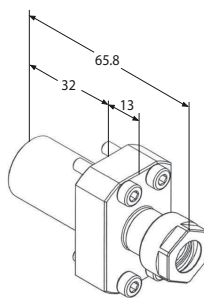
Portautensile fisso
