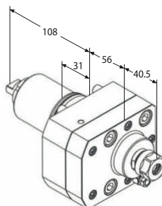
Motorizzato assiale
