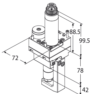
Motorizzato porta fresa a disco
