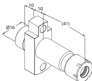
Porta punta
