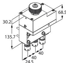
Motorizzato trasversale triplo
