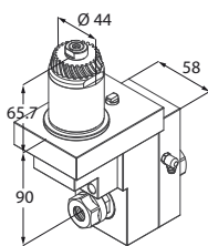
Motorizzato assiale
