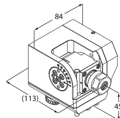
Motorizzato radiale regolabile
