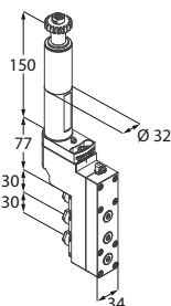
Motorizzato assiale
