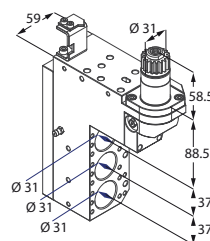
Motorizzato singolo
