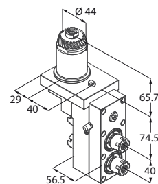
Motorizzato assiale doppio
