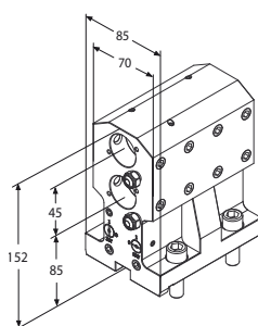
Portabareno doppio
