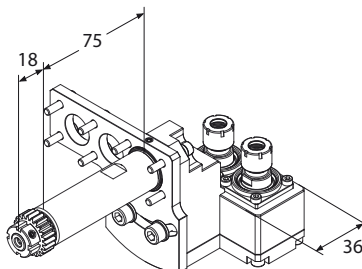
Motorizzato radiale
