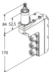
Motorizzato assiale triplo
