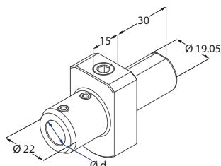
Portabareno
