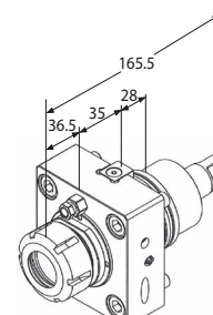
Motorizzato radiale
