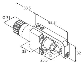
Unità portacreatore
