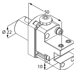
Portautensile
