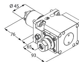
Motorizzato radiale
