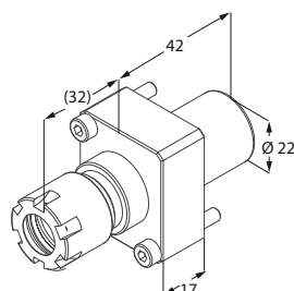
Porta punta
