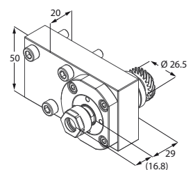
Motorizzato assiale
