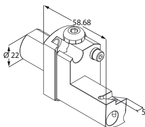
Portautensile a tornire
