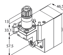
Motorizzato trasversale
