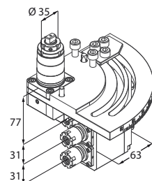
Motorizzato assiale doppio regolabile
