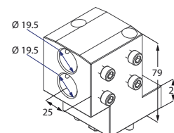
Portabareno doppio
