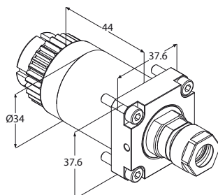
Motorizzato radiale
