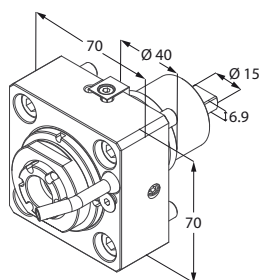
Motorizzato radiale
