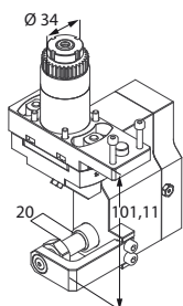
Unità portacreatore
