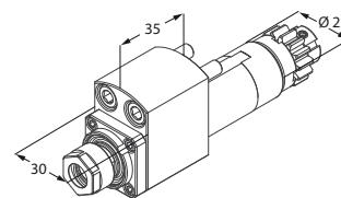
Motorizzato trasversale
