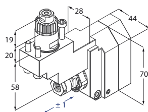
Motorizzato radiale
