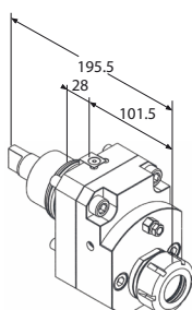
Motorizzato radiale
