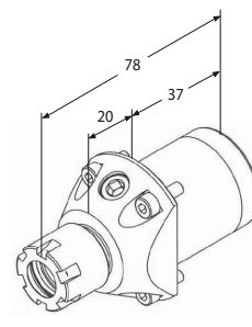
Portautensile fisso
