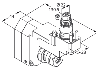
Motorizzato trasversale
