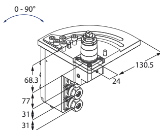
Motorizzato triplo
