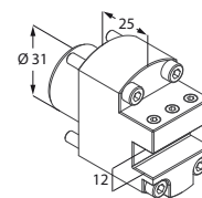
Portautensile
