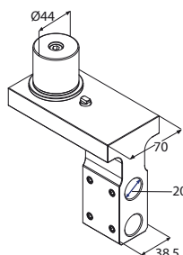
Portabareno doppio
