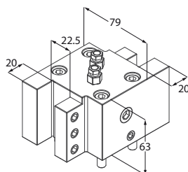
Portautensile
