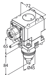
Motorizzato radiale
