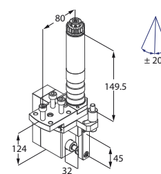
Unità portatore
