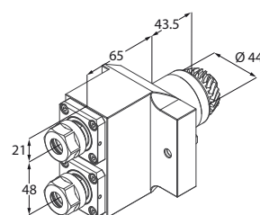
Motorizzato radiale doppio
