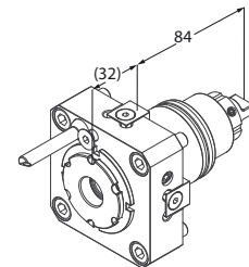
Motorizzato assiale
