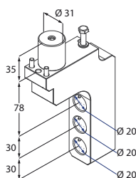
Portabareno
