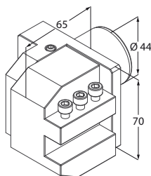
Portautensile
