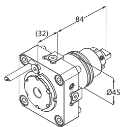
Motorizzato assiale
