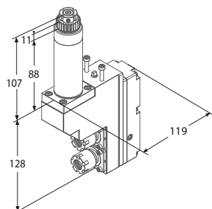
Motorizzato assiale doppio
