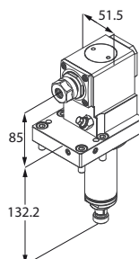
Motorizzato radiale
