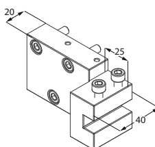
Portautensile
