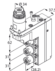
Motorizzato triplo
