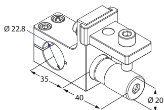
Portautensile ad aria
