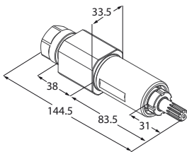
Motorizzato radiale
