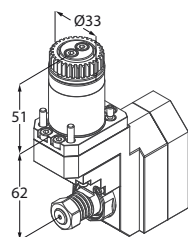
Motorizzato porta fresa a disco
