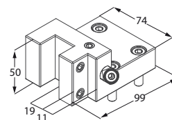
Portautensile
