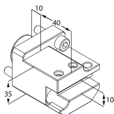
Portautensile
