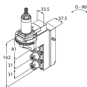
Motorizzato assiale triplo
