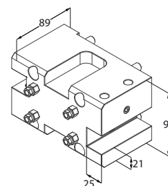
Portautensile doppio
