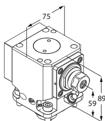
Motorizzato radiale
