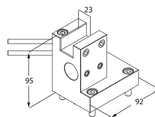
Portautensile
