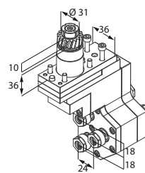
Motorizzato triplo
