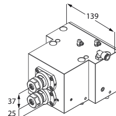
Motorizzato doppio per foratura profonda
