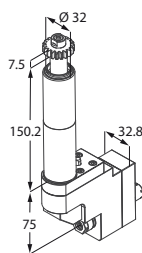
Motorizzato singolo
