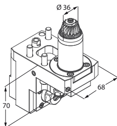
Motorizzato radiale
