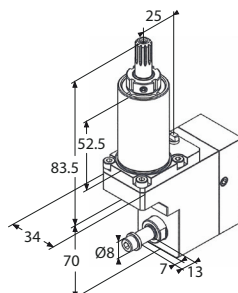
Motorizzato porta fresa a disco
