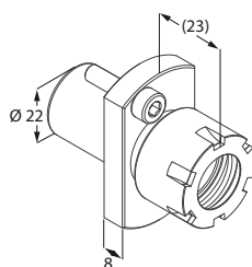
Porta punta
