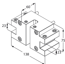
Portautensile doppio
