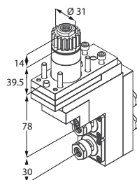
Motorizzato doppio
