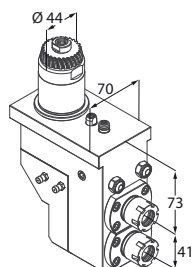
Motorizzato radiale
