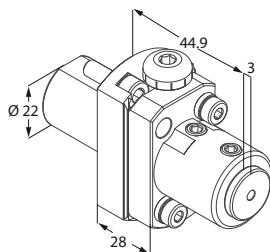
Portautensile registrabile
