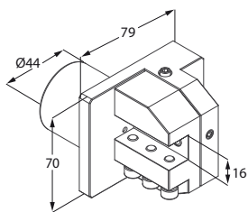
Portautensile
