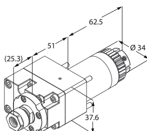
Motorizzato trasversale
