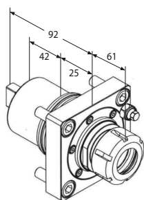
Motorizzato assiale
