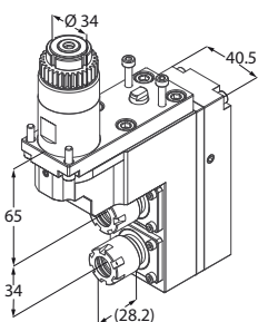
Motorizzato assiale doppio
