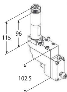
Motorizzato assiale
