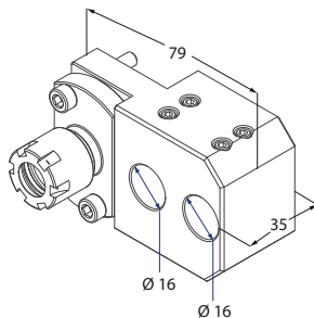
Estensione per portautensile
