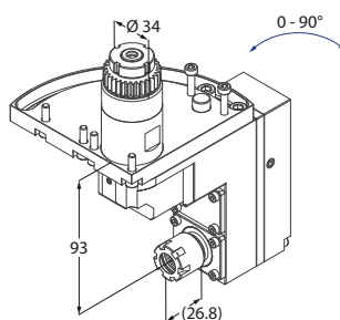
Motorizzato assiale registrabile
