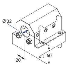
Portabareno
