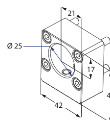
Porta punta
