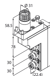
Motorizzato triplo
