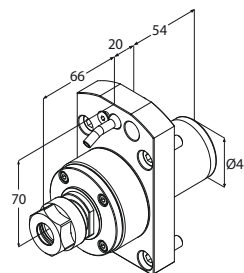
Motorizzato radiale
