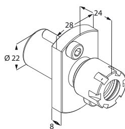
Porta punta
