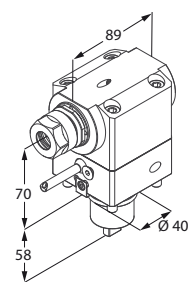
Motorizzato radiale
