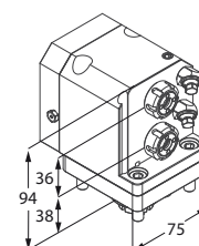
Motorizzato radiale
