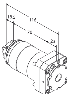
Motorizzato porta fresa
