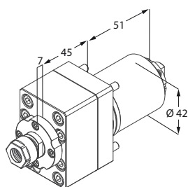
Motorizzato singolo
