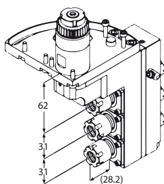
Motorizzato assiale triplo
