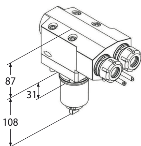
Motorizzato radiale
