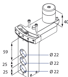
Portautensile ad aria
