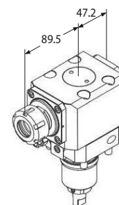
Motorizzato radiale
