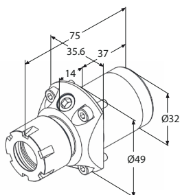
Portautensile fisso
