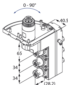
Motorizzato triplo
