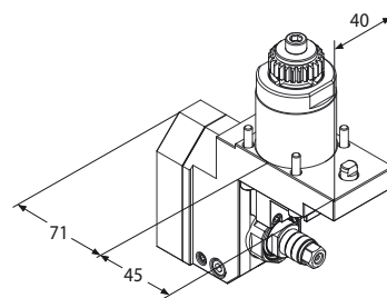
Portafresa a disco
