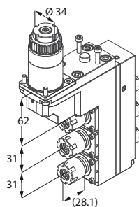
Motorizzato triplo
