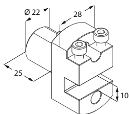
Portautensile
