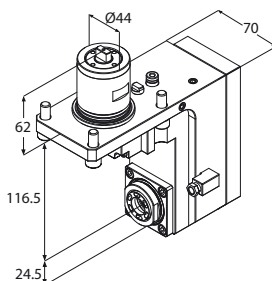
Motorizzato assiale
