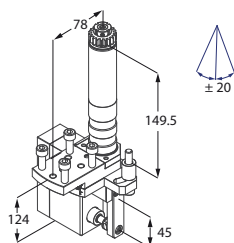
Unità portatore
