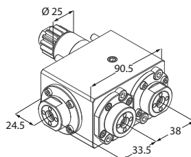
Motorizzato radiale e assiale
