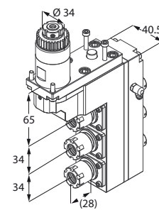
Motorizzato triplo
