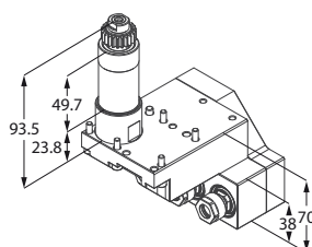
Motorizzato triplo
