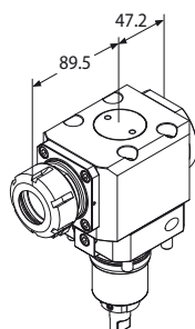
Motorizzato radiale
