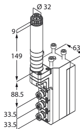
Motorizzato triplo
