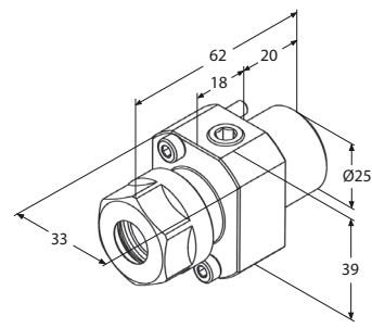
Portapinza fisso con refrigerazione interna
