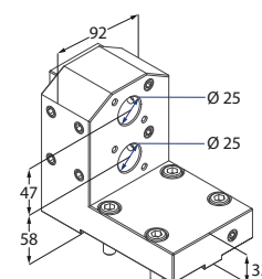
Portabareno disassato
