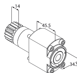
Motorizzato porta fresa
