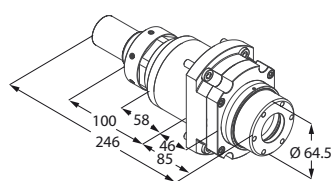
Motorizzato senza bussola di guida
