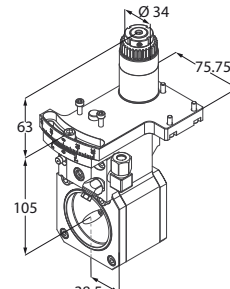
Tourbillonnage
