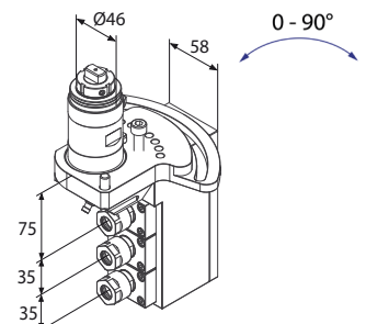
Motorizzato assiale triplo regolabile
