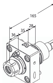
Motorizzato radiale
