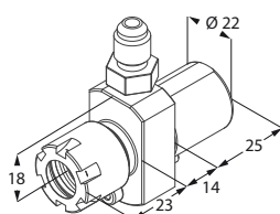
Porta punta
