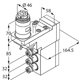
Motorizzato triplo
