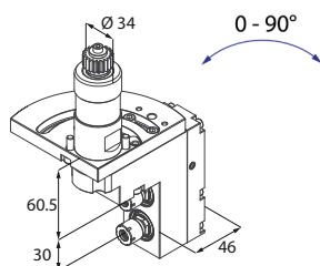
Motorizzato assiale doppio regolabile
