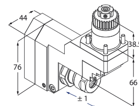
Motorizzato radiale e assiale
