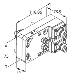
Motorizzato assiale
