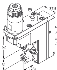
Motorizzato doppio
