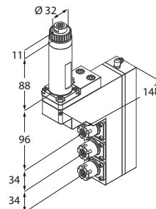
Motorizzato assiale triplo
