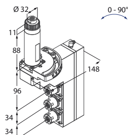
Motorizzato assiale triplo
