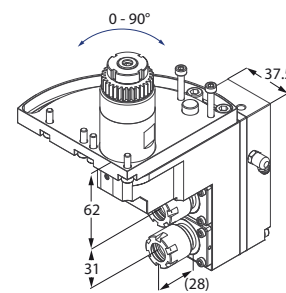
Motorizzato doppio
