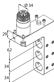
Portabareno
