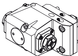
Motorizzato radiale
