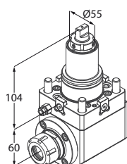
Motorizzato radiale
