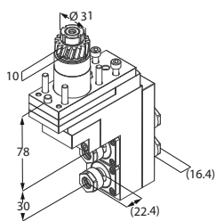
Motorizzato doppio
