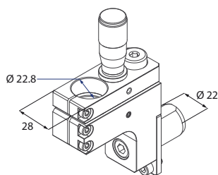
Portautensile ad aria
