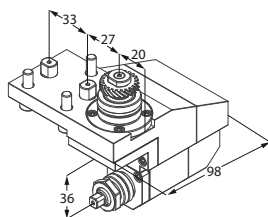
Motorizzato porta fresa
