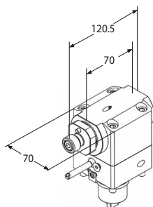
Poligonatore
