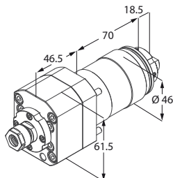
Motorizzato trasversale
