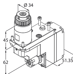
Motorizzato radiale e assiale
