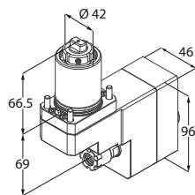
Motorizzato radiale
