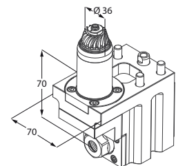
Motorizzato radiale
