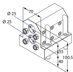
Portabareno doppio
