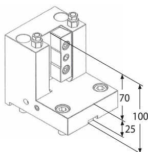
Portautensile
