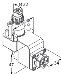
Motorizzato trasversale
