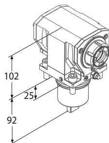
Motorizzato assiale
