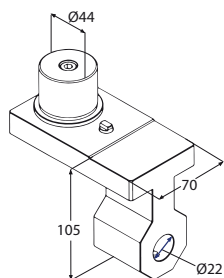
Portabareno
