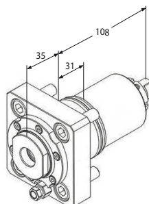
Motorizzato assiale
