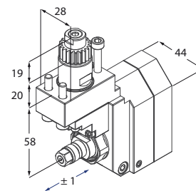
Motorizzato porta fresa a disco
