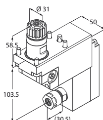
Motorizzato trasversale
