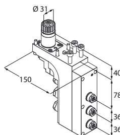
Motorizzato assiale triplo fronte/retro
