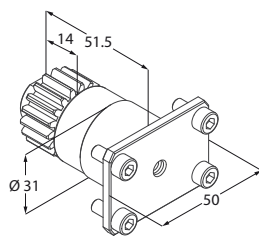
Unità di rinvio
