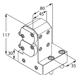
Portabareno
