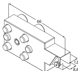
Portautensile a tornire
