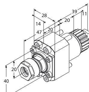
Motorizzato radiale e assiale
