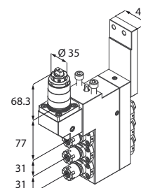
Motorizzato triplo
