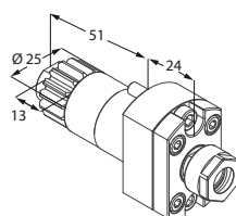
Motorizzato singolo
