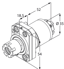
Motorizzato singolo
