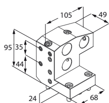
Portabareni
