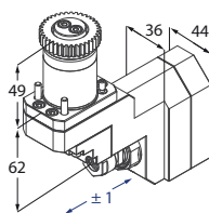
Motorizzato radiale e assiale
