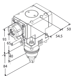
Motorizzato assiale
