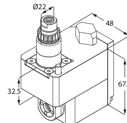
Motorizzato trasversale
