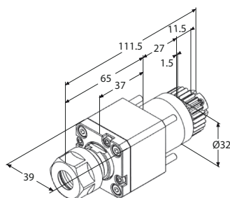
Motorizzato radiale e assiale
