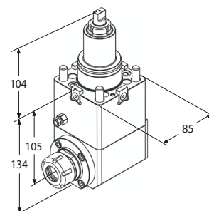
Motorizzato assiale
