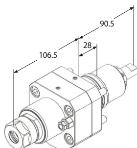
Motorizzato assiale
