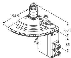
Motorizzato doppio
