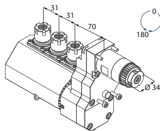
Motorizzato triplo
