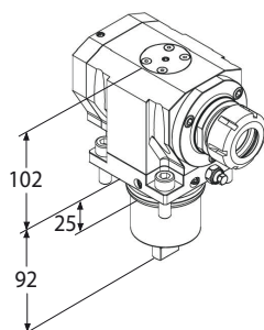
Motorizzato assiale
