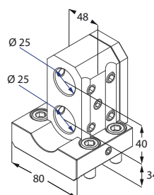
Portabareno doppio
