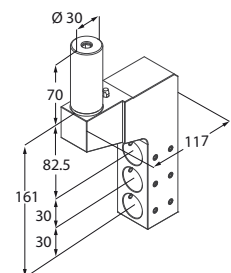
Portabareno triplo
