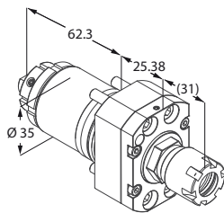
Motorizzato singolo
