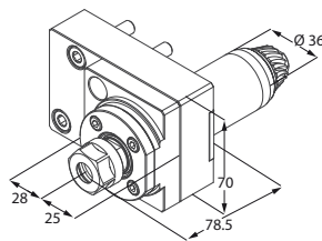
Motorizzato assiale
