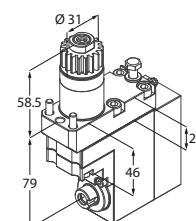
Unità poligonale
