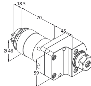
Motorizzato trasversale
