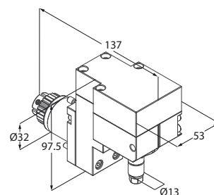
Motorizzato portafresa
