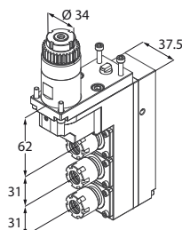
Motorizzato assiale triplo
