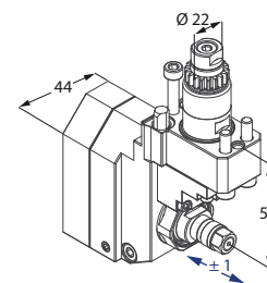
Motorizzato porta fresa
