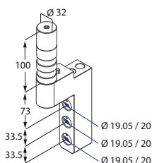
Portabareno
