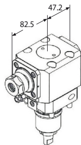
Motorizzato radiale
