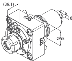
Motorizzato assiale
