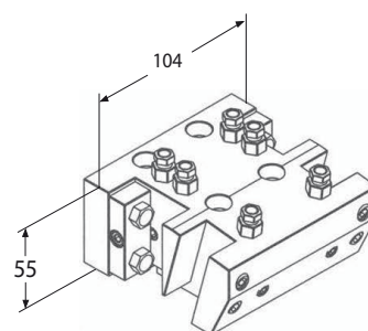
Portautensile
