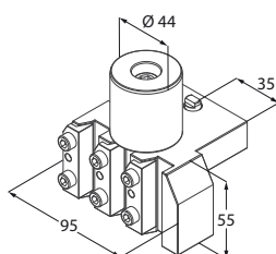
Portautensile triplo
