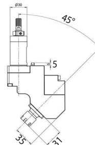
Motorizzato assiale
