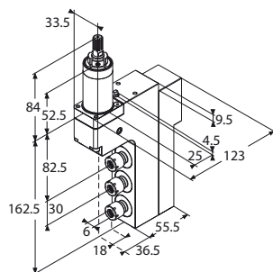
Motorizzato assiale triplo
