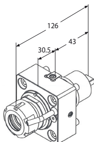
Motorizzato radiale
