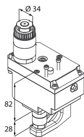
Motorizzato porta fresa
