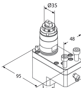
Motorizzato assiale
