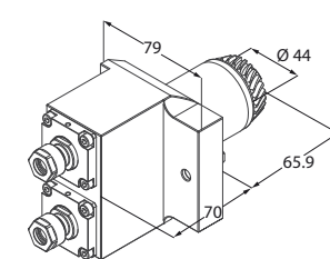
Motorizzato radiale doppio
