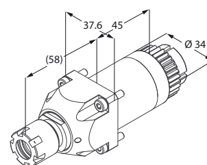
Motorizzato trasversale
