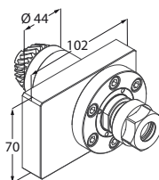
Motorizzato radiale
