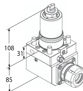
Motorizzato radiale
